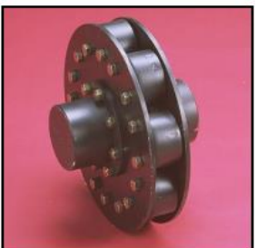
SNA-NG (Barracuda) 扭力 800 KN*m, 角度10 deg 偏移 (3 directions) +/- 50 mm
